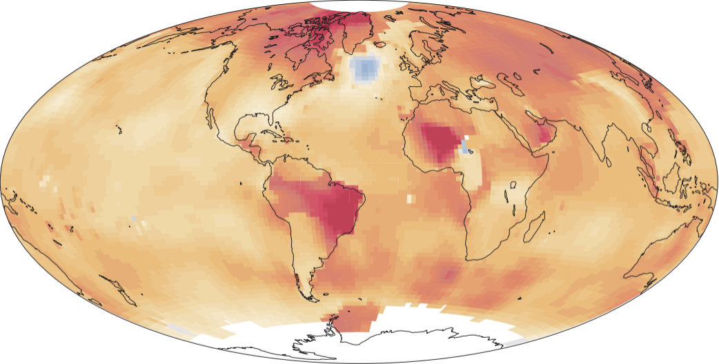
Linear temperature trend, °C per century
