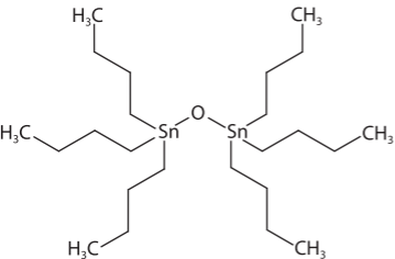
Tributyl tin (TBT)
