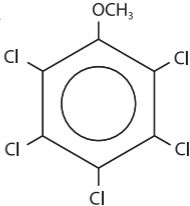
PCA
