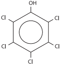
PCP
